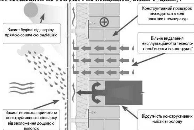
Рис. 1. Ефект термосу вентильованого фасаду
