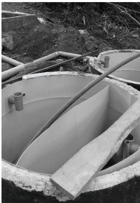
Рис. 2. Монтаж полімерних конструкцій в існуючих бетонних стінках очисних споруд
