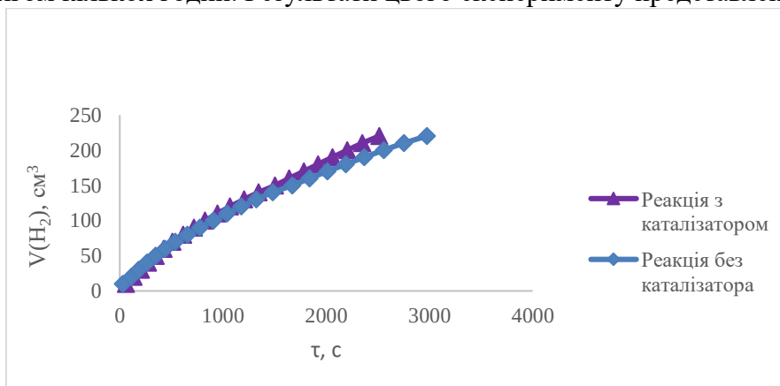
Рис. 1. Залежність об'єму виділеного водню від тривалості реакції гідролізу \text{NaBH}_4 за кімнатної температури
